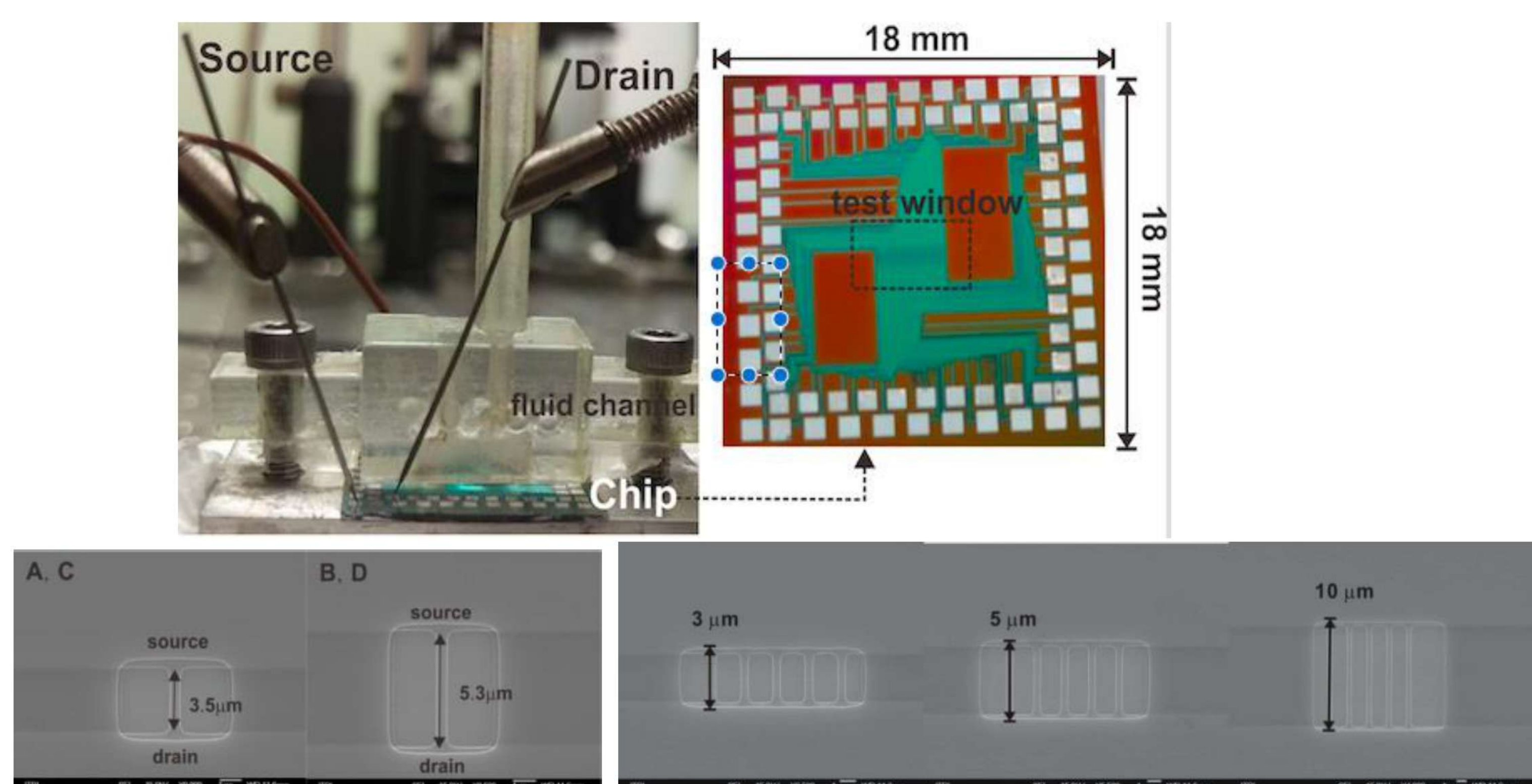
奈米線氯化鈉/葡萄糖濃度感測晶片與量測系統
