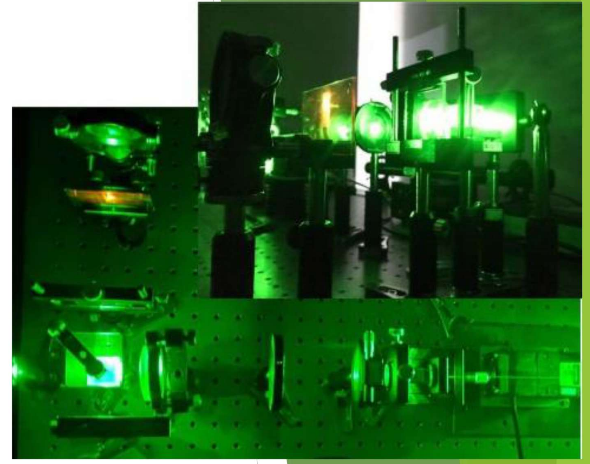
全像式感測器拍攝系統
