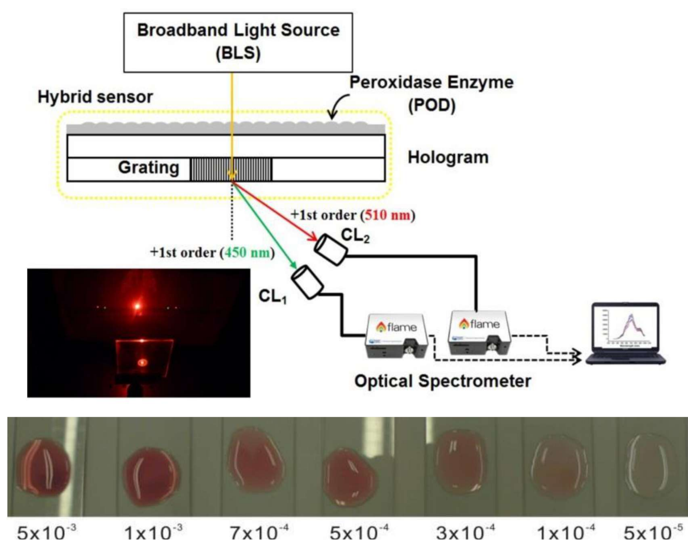
複合式(全像光柵/POD酵素) H_2O_2 感測系統
