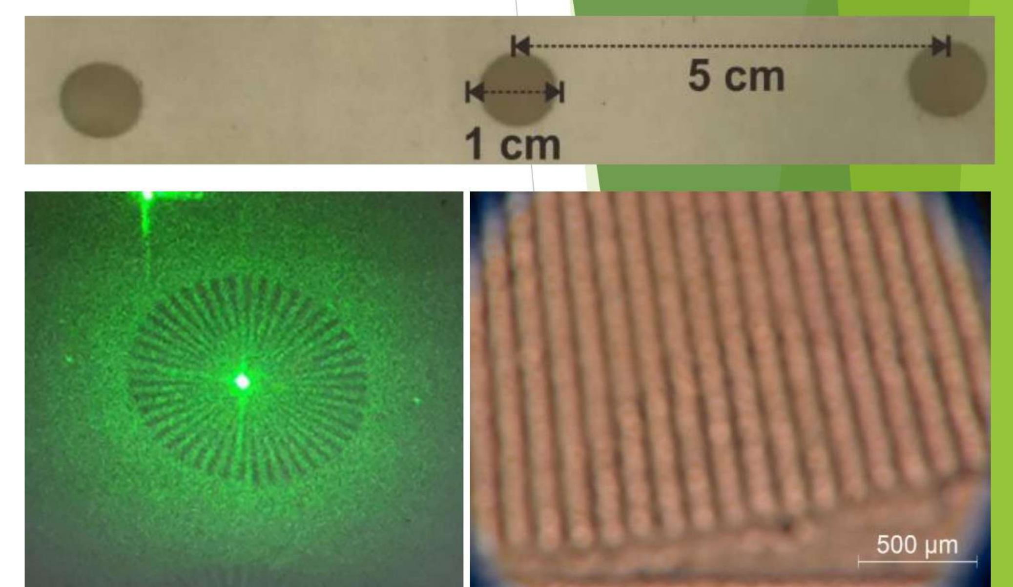
線性/旋轉角全像式感測器
