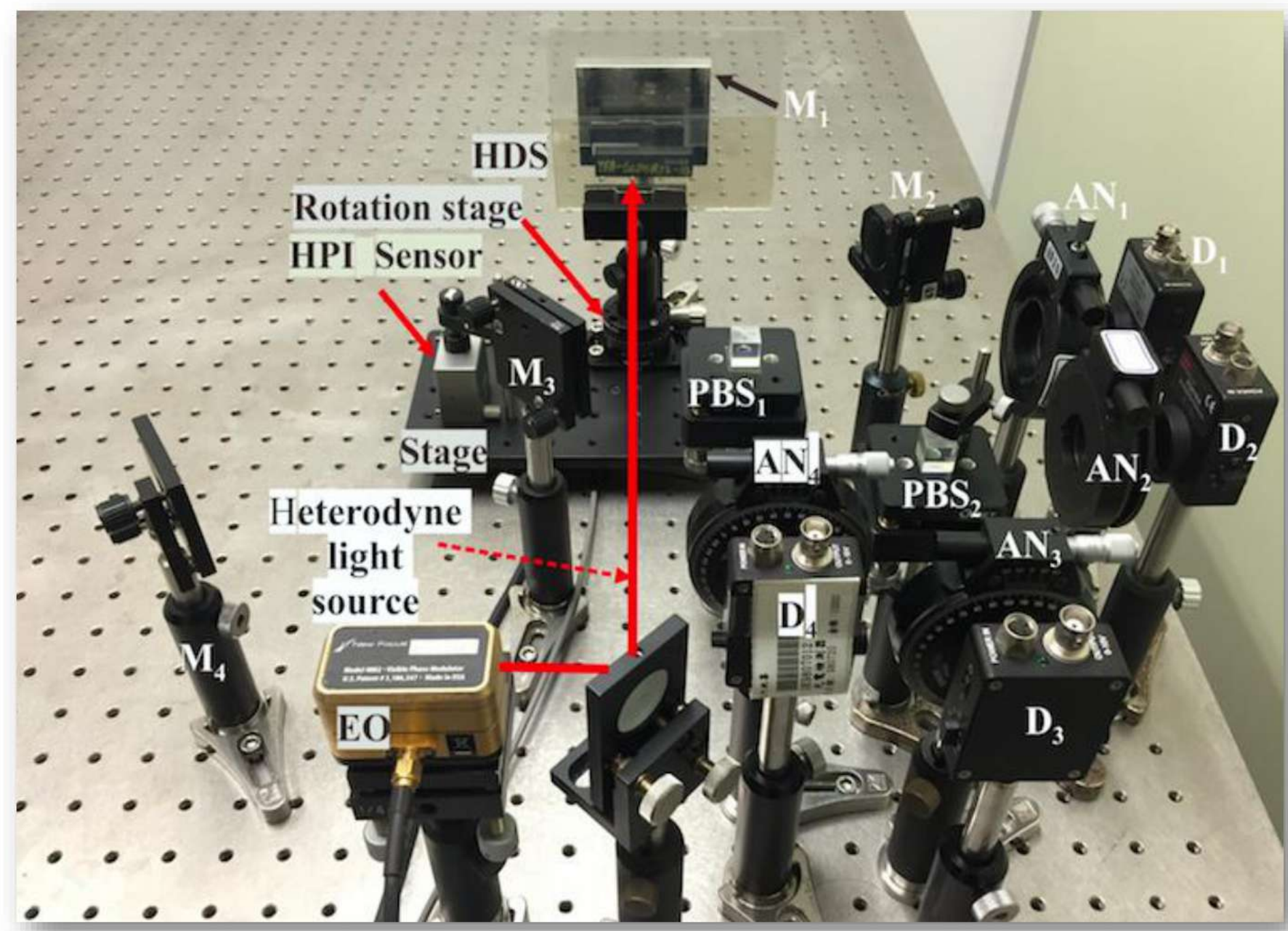
線性位移監控系統
