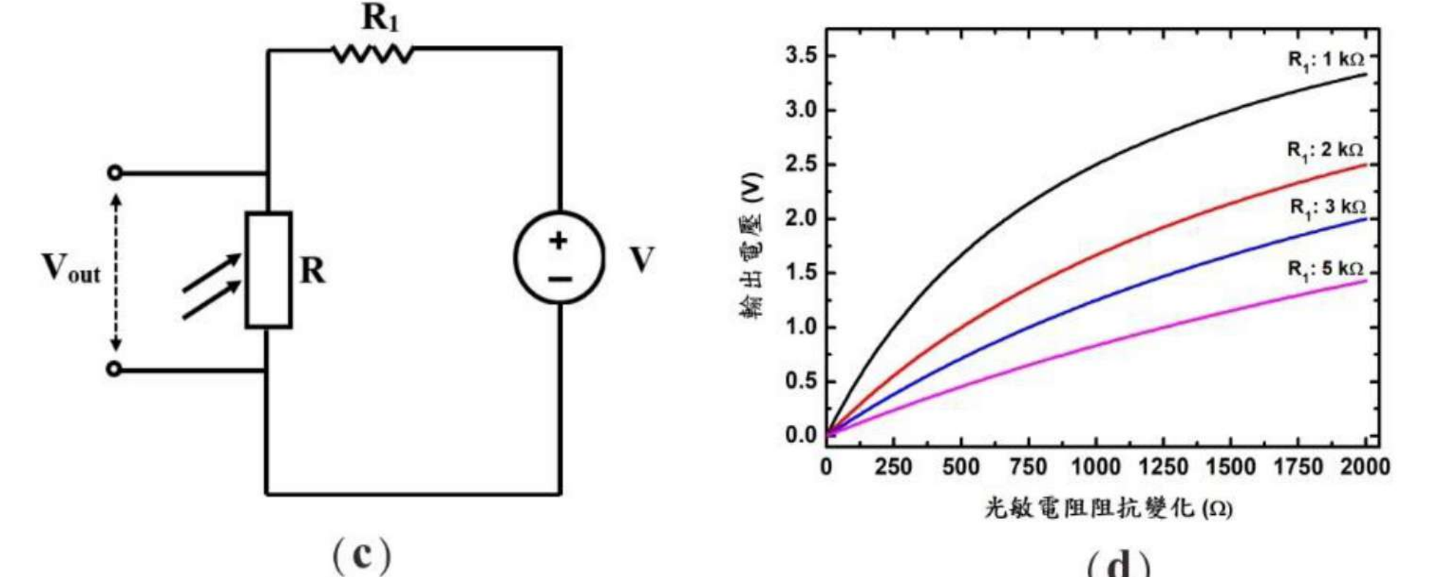
嵌入式介面活性劑濃度感測系統
