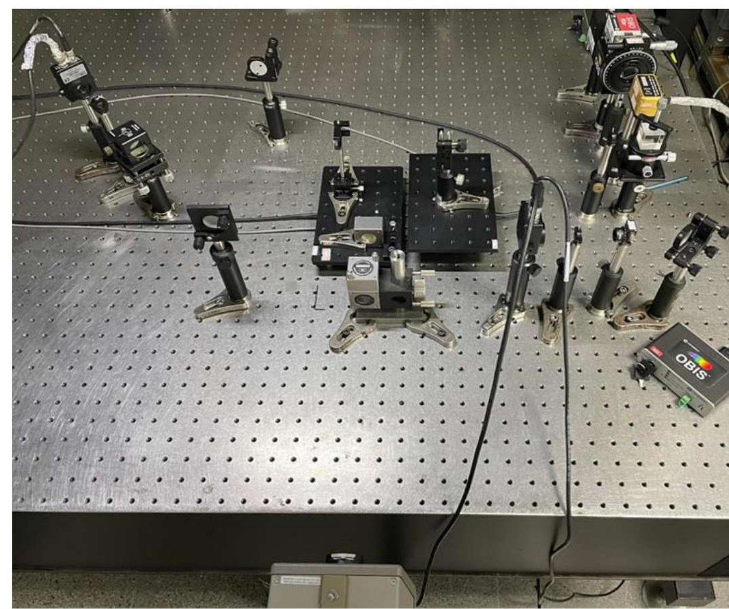
光柵週期量測系統
